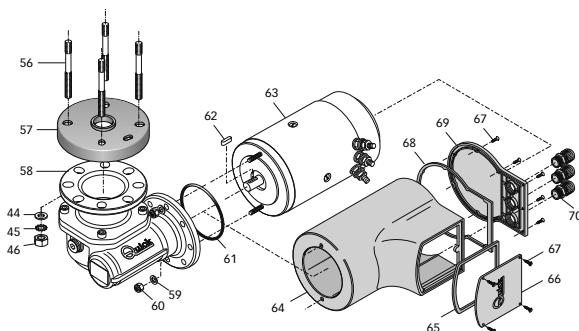
MOTORIDUTTORE 700/1000W
