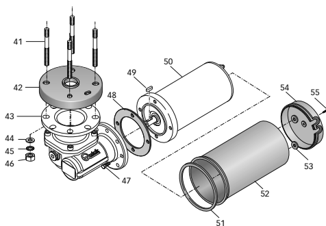
MOTORIDUTTORE 300/500W
